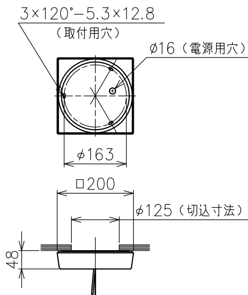
取付板部詳細 S:1/10
